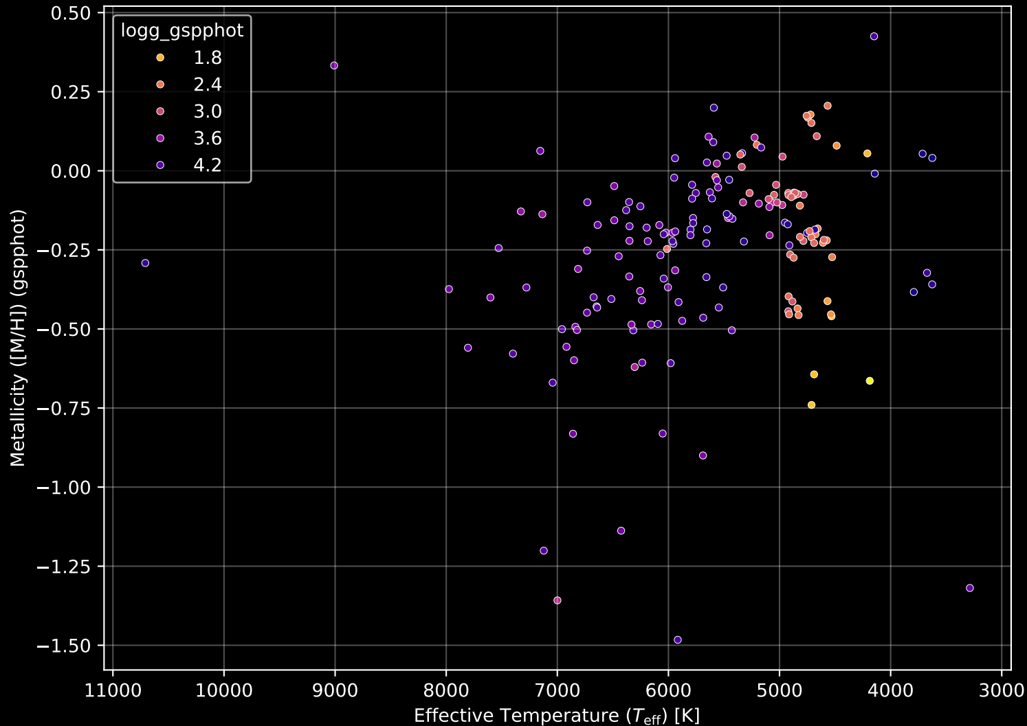
APOGEE DR17 Field: [CVZ_OB07_btx] Stellar Population Parameters (n= 173)
